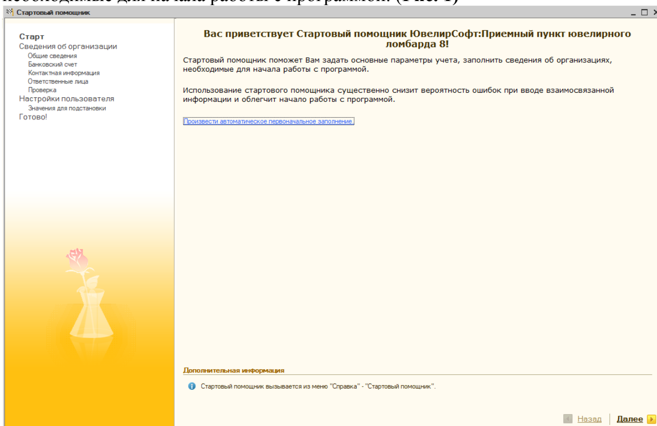
Рисунок 1. Стартовый помощник
